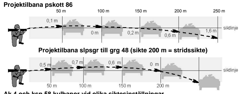
Ak 4 och ksp 58 kulbanor vid olika siktesinställningar
